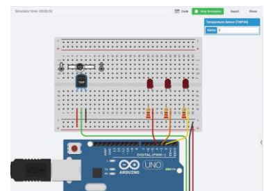
Tinkercad Circuits
